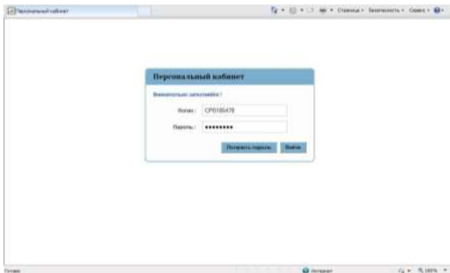
Рис. 1. Авторизация пользователя.
